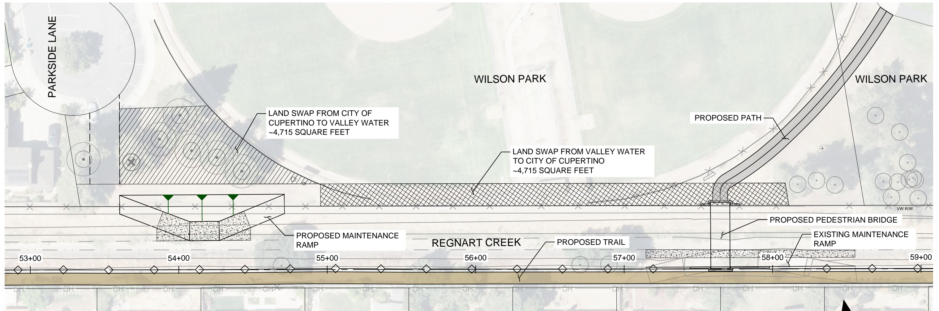
PLAN SCALE: 1" = 40'
